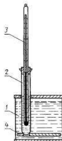
1 — масляная баня; 2 — стеклянная пробирка; 3 — термометр; 4 — металлический диск
